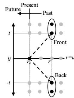
FIG. 11. t vs. r
